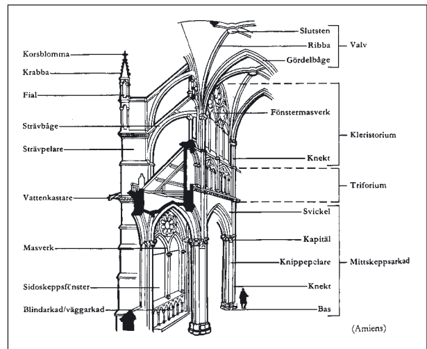
Den principiella uppbyggnaden av en gotisk katedral och olika utsmyckningsdetaljer.
