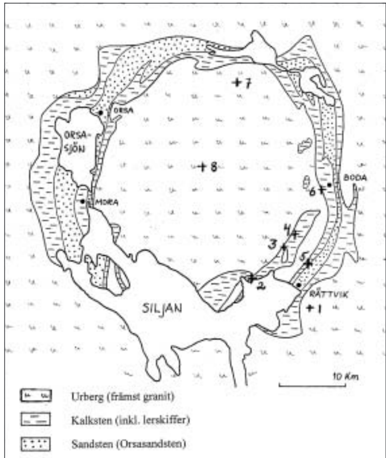
Berggrunden i Siljansringen samt beskrivna platser (1-8).
